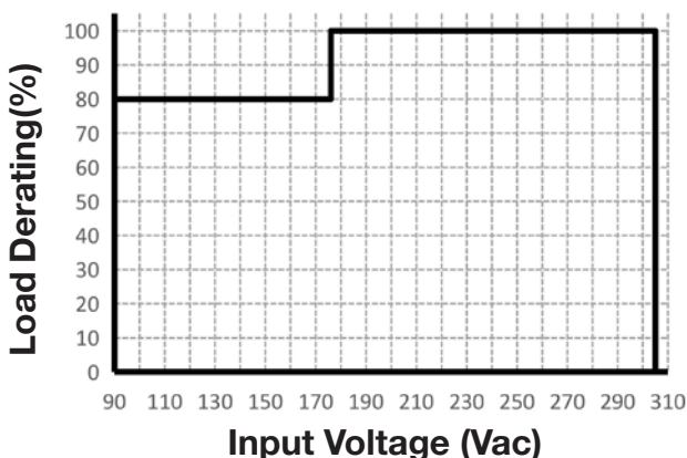
Tensión de entrada y temperatura vs. reducción de carga / Input Voltage and Temperature vs. Load Derating / Tension d'entrée et température vs. réduction de charge
