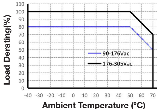
Tensión de entrada y temperatura vs. reducción de carga / Input Voltage and Temperature vs. Load Derating / Tension d'entrée et température vs. réduction de charge
