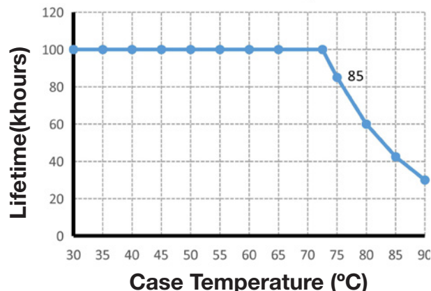
Vida útil vs. temperatura de la carcasa / Lifetime vs. Case Temperature / Durée de vie vs. température du boîtier
